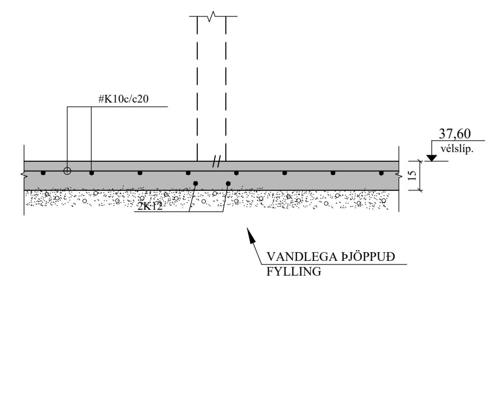
B2 SNIÐ. 1:20 1-02 Innveggur.
