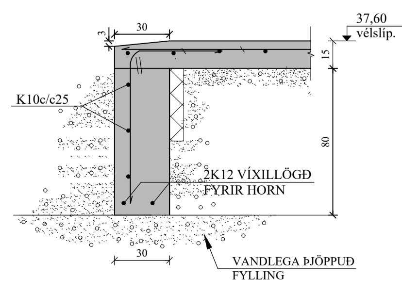
C2 SNIÐ. 1:20 1-02
