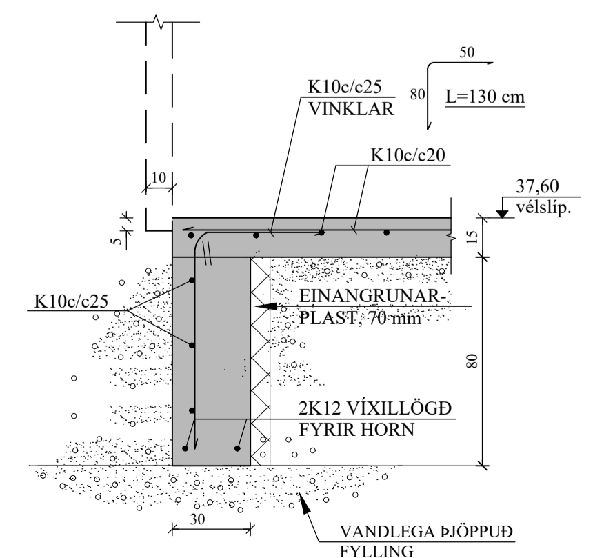
A2 SNIÐ. 1:20 1-02
